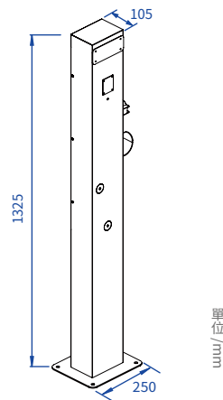
充電樁立柱 (簡易型)
