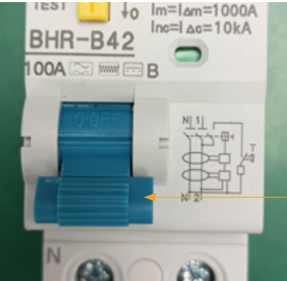
漏電斷路器
